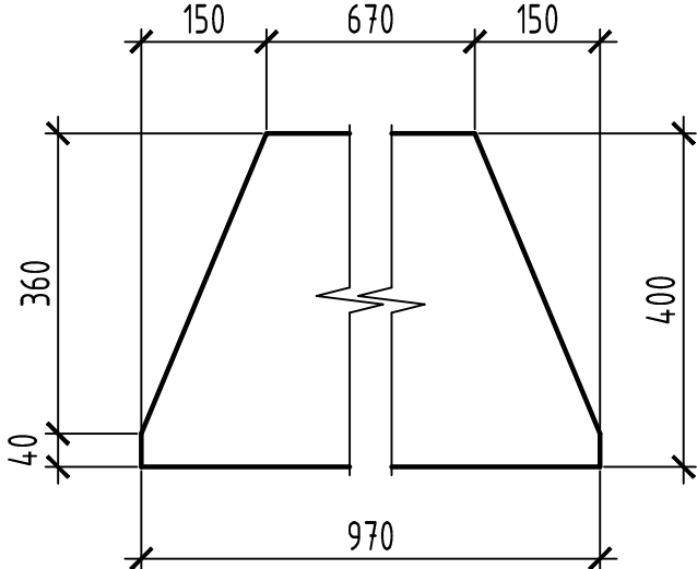
поз.24 (M1:10) 96 шт. 502006941C2459
