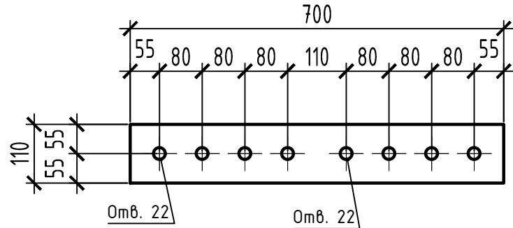
поз.27 (M1:10) 48 шт. 12041062001C2459
