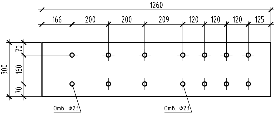
поз.38 (M1:10) 8 шт. 12029561851C2459
