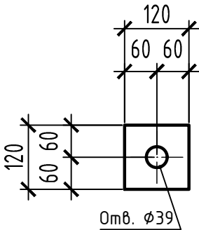
поз.24 (M1:10) 96 шт. 502006941C2459
