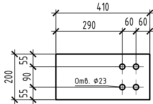
поз.27 (M1:10) 48 шт. 12041062001C2459
