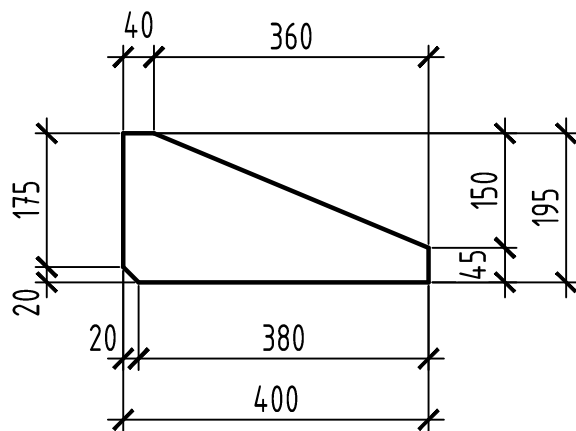
поз.26 (M1:10) 56 шт. 12070061101C2459
