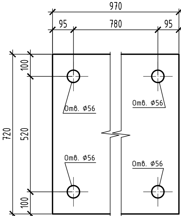
поз.37 (M1:10) 14 шт. 200126063001C2459
