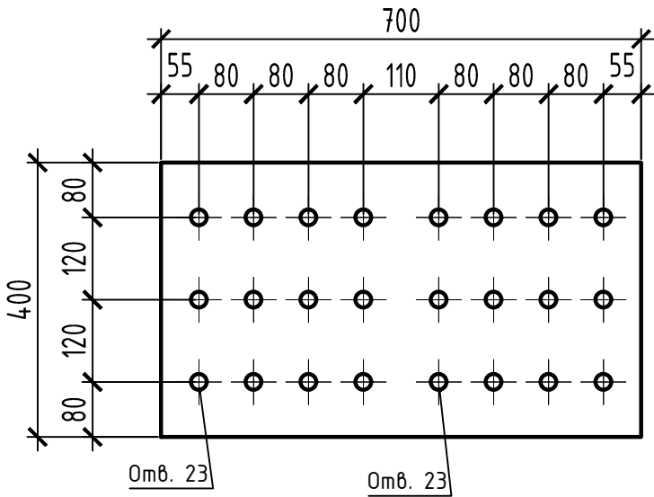
поз.34 (M1:10) 16 шт. 12026761401C2459
