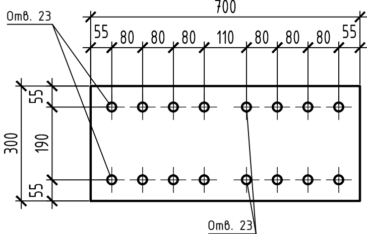
поз.32 (M1:10) 28 шт. 12070063001C2459
