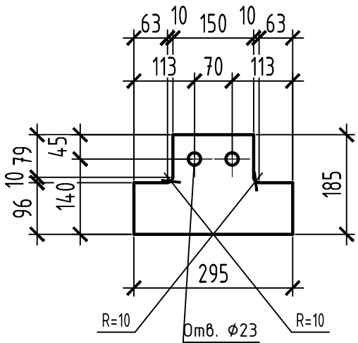
поз.30 (M1:10) 28 шт. 14040061961C2459
