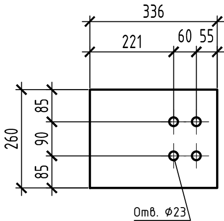
поз.39 (M1:10) 8 шт. 12033662601C2459
