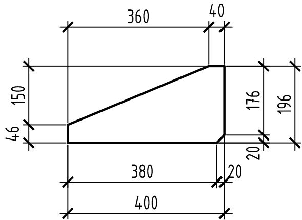
поз.31 (M1:10) 28 шт. 14097064001C2459
