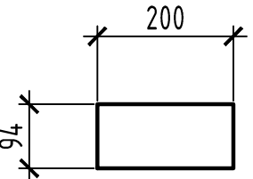
поз.25 (M1:10) 56 шт. 14040061951C2459
